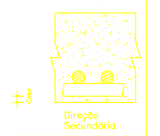
Detalhe genérico do abojamento de armaduras positivas
